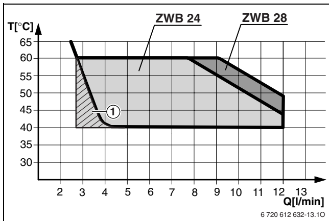
Sl. 12 Diagram za vstopno temperaturo hladne vode +15 °C.
