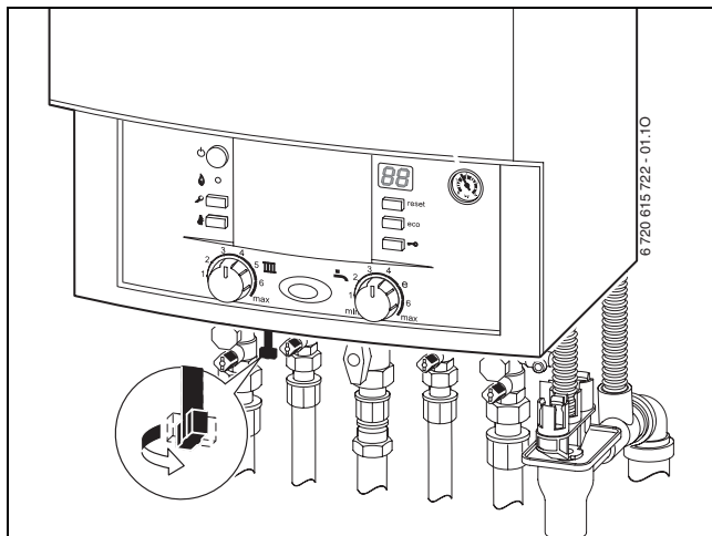
Sl. 6 Navpična montažna plošča
